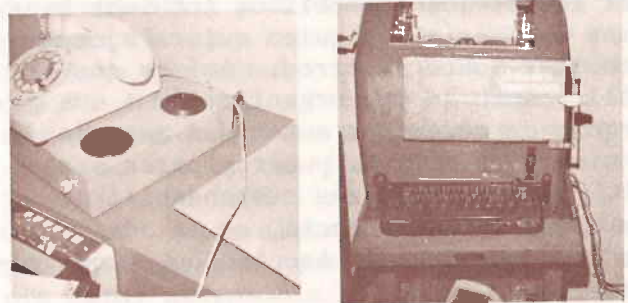
El adaptador (izquierda) permite enviar por teléfono los mensajes escritos en T.T.Y. (derecha).
